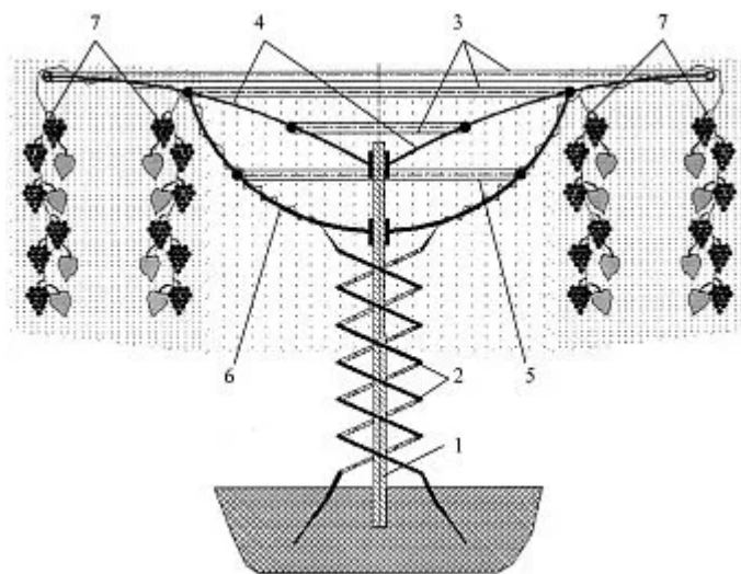
Чертёж т-образной опоры
