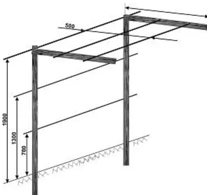
Чертёж г-образной шпалеры
